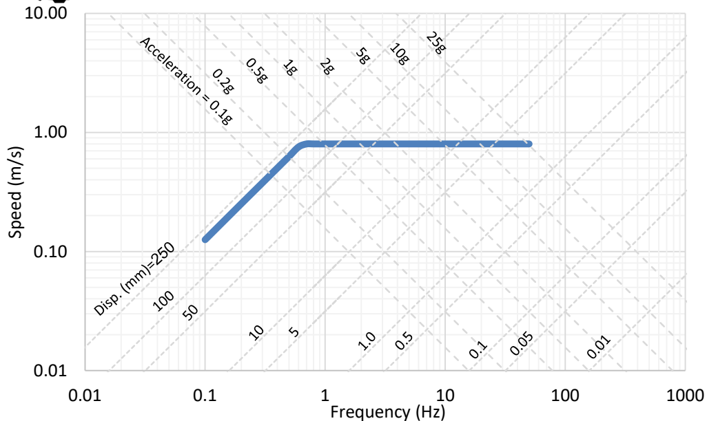
نمودار عملکرد اکچویاتور آزاد در سرعت 1 متر بر ثانیه
