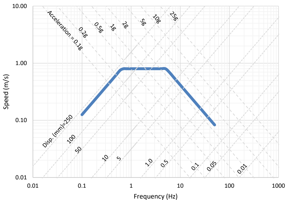
نمودار عملکرد اکچویاتور تحت اثر 20 تن نیرو و سرعت 1 متر بر ثانیه
